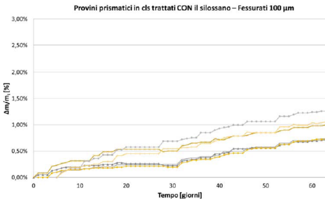
Figura 7: variazione % in peso – provini fessurati a 100 µm trattati con PROTECH
