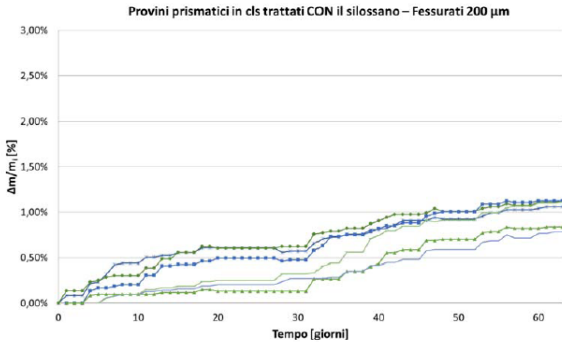
Figura 9: variazione % in peso – provini fessurati a 200 μm trattati con PROTECH
