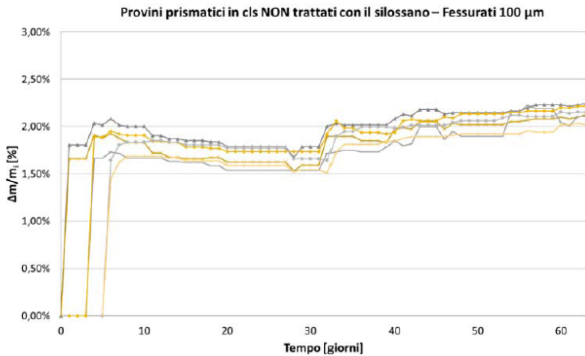
Figura 6: variazione % in peso – provini non trattati fessurati a 100 µm
